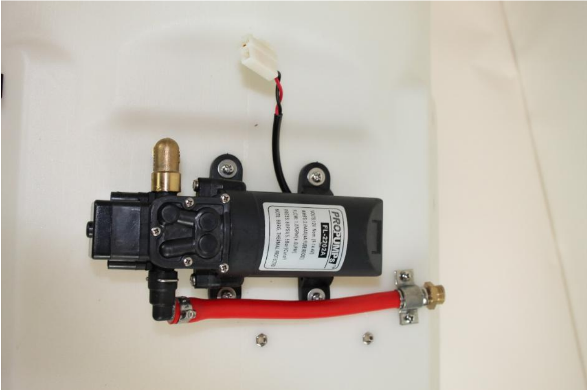
Kobling til pumpe fra batteriet
